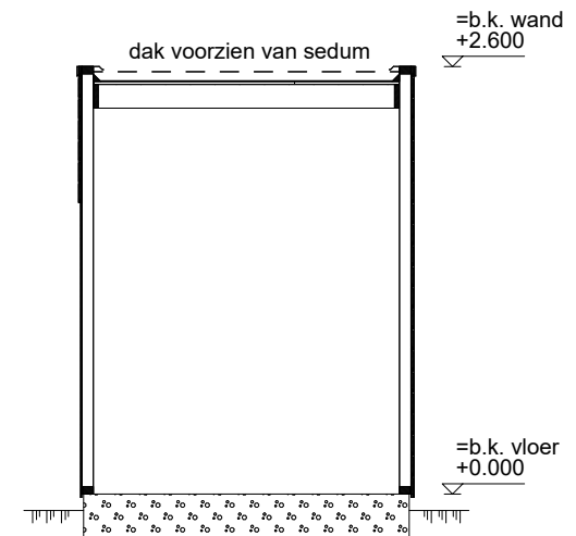
DOORSNEDE
