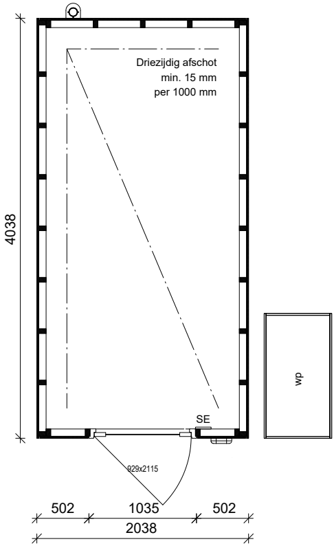
PLATTEGROND (Tuinzijde)
