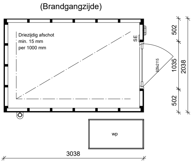
PLATTEGROND (Tuinzijde)
