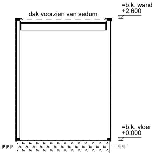
DOORSNEDE
